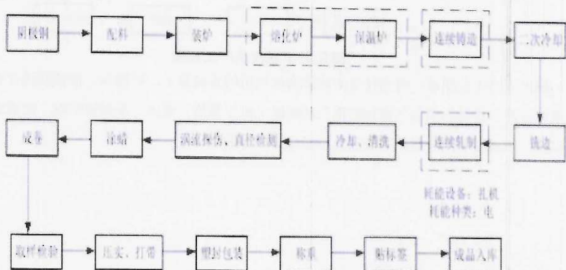
图 3.1-4 工艺流程图
